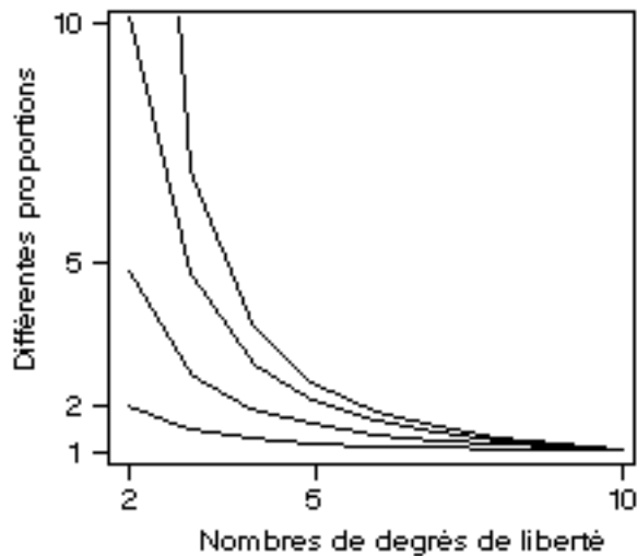
Figure 1. Représentation graphique des proportions des colonnes (3), (6) et (9) du tableau 1, et des résultats correspondants relatifs aux variances, pour 2 à 10 degrés de liberté: les différentes lignes brisées concernent respectivement, de haut en bas, les estimations de variances, les tests d'égalité de deux moyennes, les estimations d'écart-types et les estimations de moyennes ou de fonctions linéaires de moyennes.
