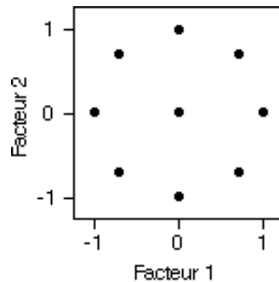
Figure 2. Positions des neuf points expérimentaux dans le cas envisagé pour deux facteurs.
